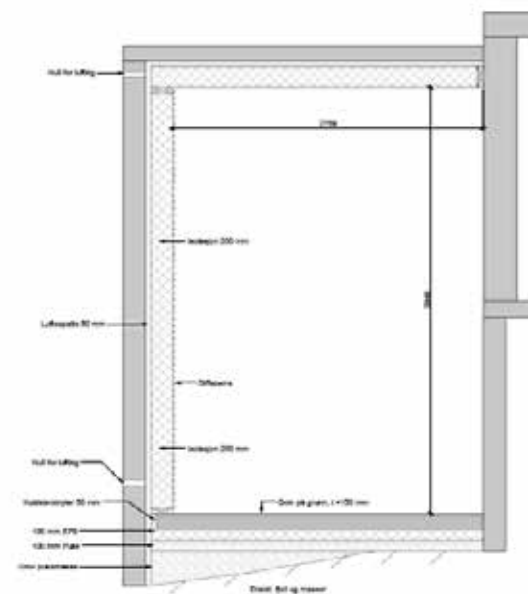
Snitt Teknisk rom/kulvert 1:20
